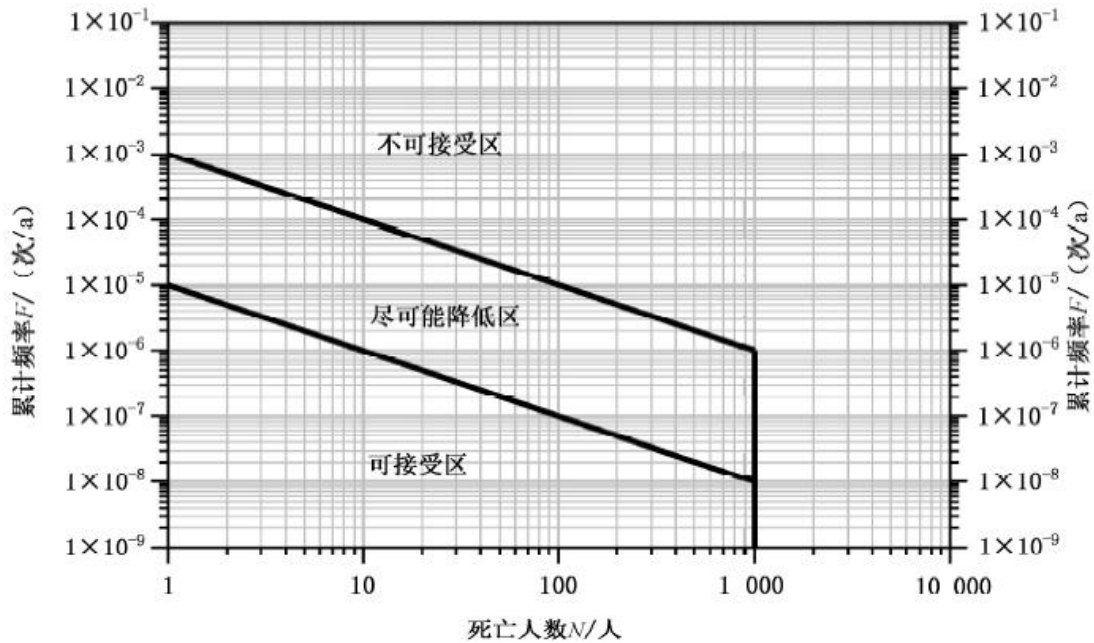
图 4.1-1 社会风险基准
