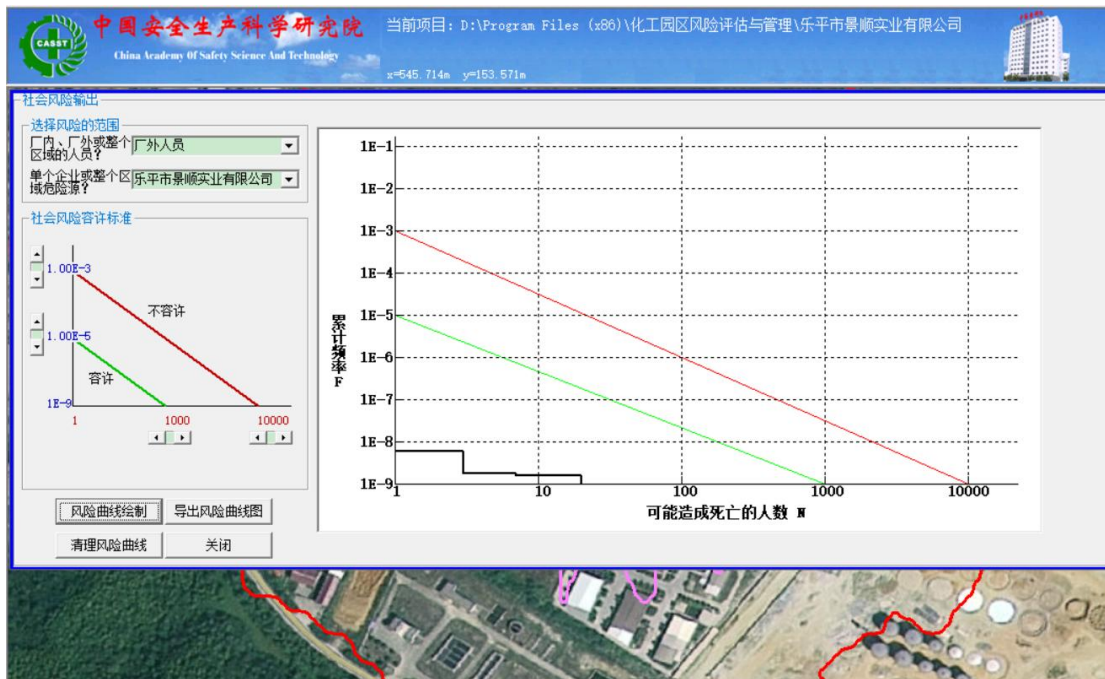
图 4.1-3 社会风险分析效果图
