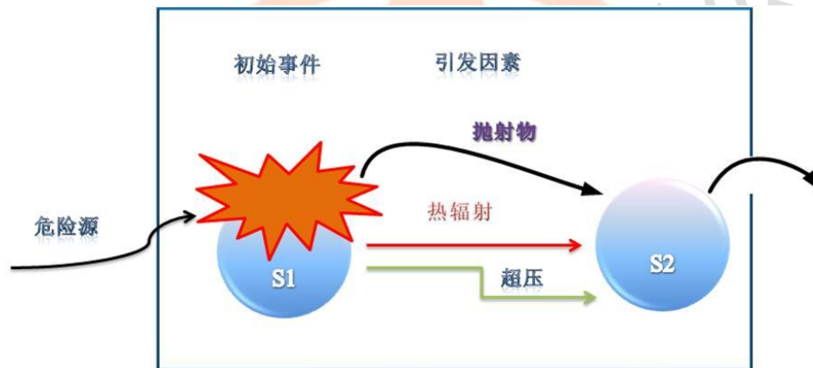
图 4.1-4 多米诺效应系统图
