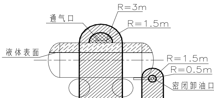
汽油的油罐车和密闭卸油口爆炸危险区域划分图
