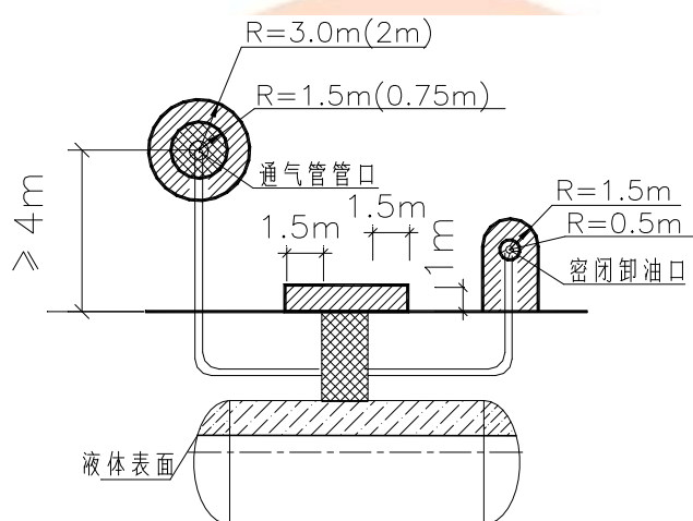
埋地卧式汽油储油罐爆炸危险区域划分图
